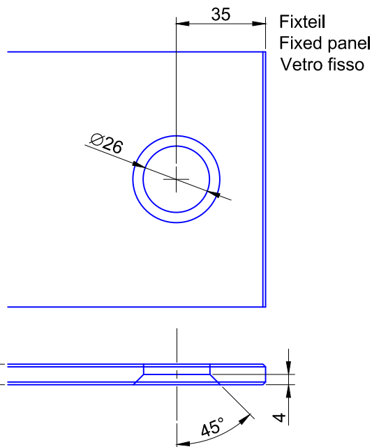
Beidseitig 90° Öffnend Türband Glas-Glas Glass-glass double sided 90° opening hinge Cerniera vetro-vetro apertura 90° interna ed esterna
