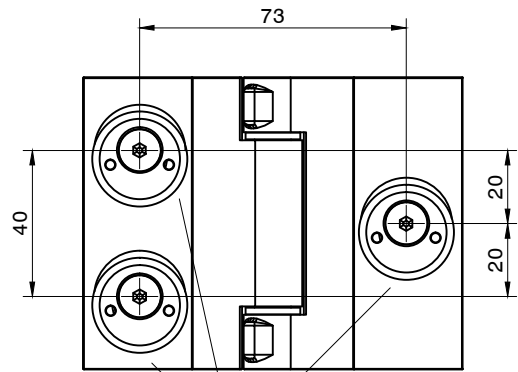
2,5mm exzentrische Einstellbolzen 2,5mm eccentric adjusting bolts Borchie eccentriche di regolazione 2,5mm
